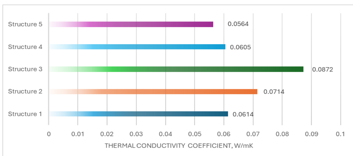
Fig. 24. Valori medii ale coeficientului de conductivitate termică pentru întregul ciclu de testare (according to Brenci et al. 2018)
